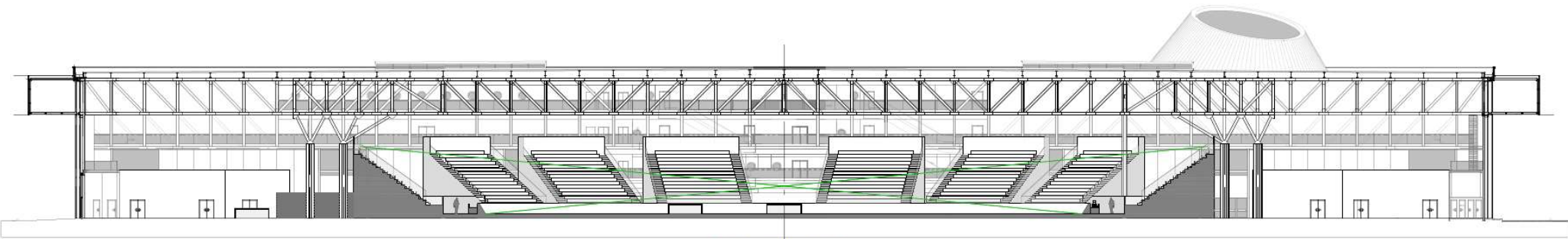
SEZIONE TRASVERSALE CON VISTA LATO SUD
