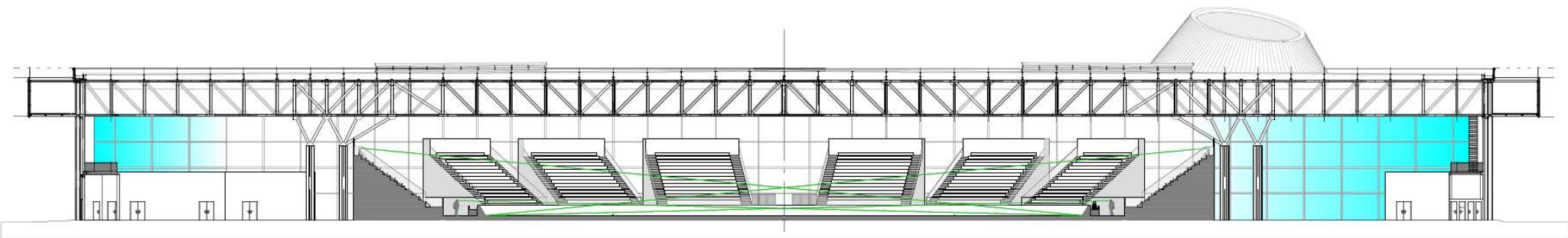
SEZIONE TRASVERSALE CON VISTA LATO NORD
