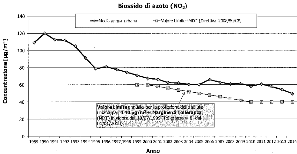
Figura 3.6 Andamento storico delle concentrazioni medie annue di NO 2 (Fonte: ARPA Lombardia 2015)
