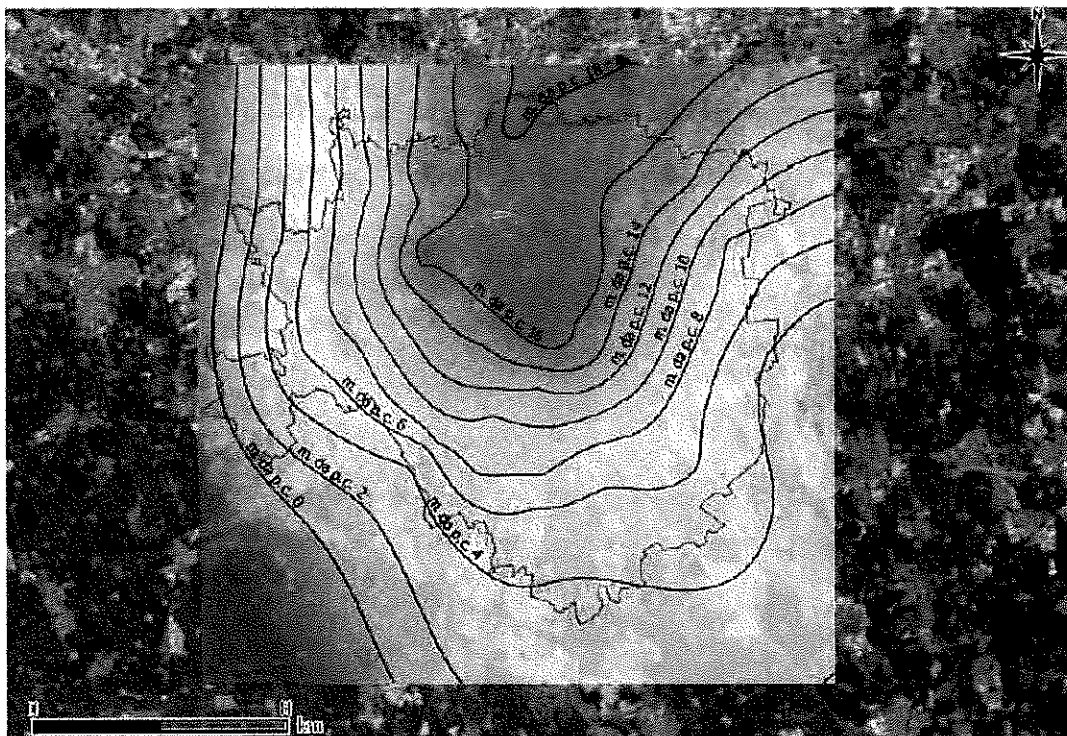
Figura 3.19 Mappa della soggiacenza ricavata dalle misure del giugno 2013
