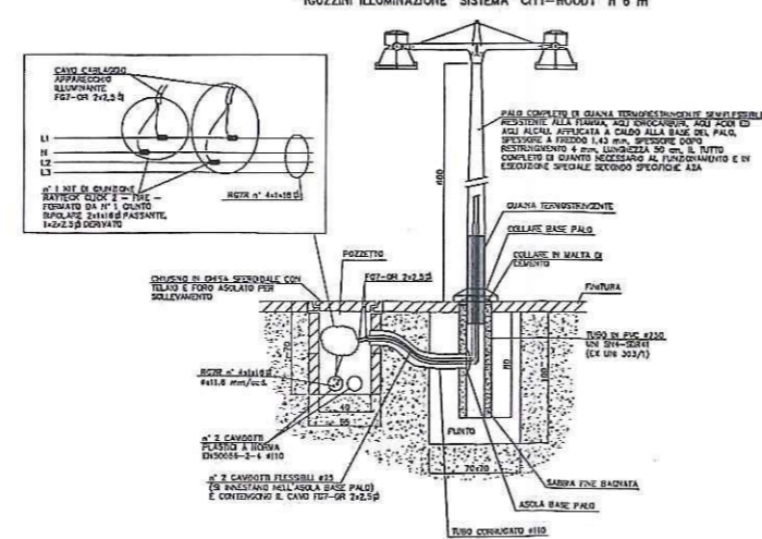
TIPICO INDICATIVO INSTALLAZIONE APPARECCHIO ILLUMINANTE "GUZZINI ILLUMINAZIONE" SISTEMA "CITY-WOODY" h 6 m
