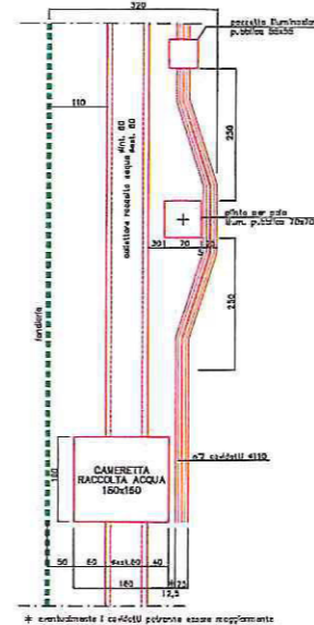
PARTICOLARE COORDINATO POSIZIONAMENTO RECIPROCO IMPIANTO DI RACCOLTA ACQUE CON IMPIANTO DI ILLUMINAZIONE PUBBLICA PLUMBI E POZZETTI IMP. LP. SOTTO SPALATI RISPETTO A CAMERETTE RACCOLTA ACQUE
