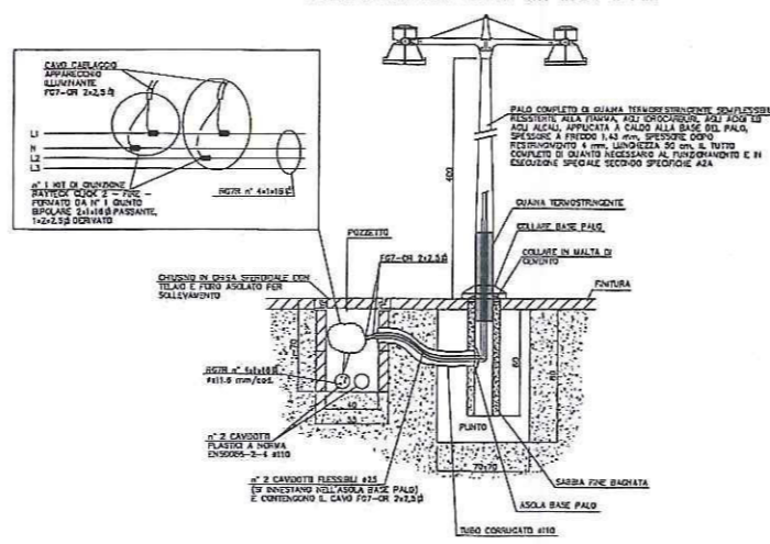
TIPICO INDICATIVO INSTALLAZIONE APPARECCHIO ILLUMINANTE "GUZZINI ILLUMINAZIONE" SISTEMA "CITY-WOODY" h 4 m
