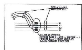
TIPICO INDICATIVO DERIVAZIONE IN POZZETTO
