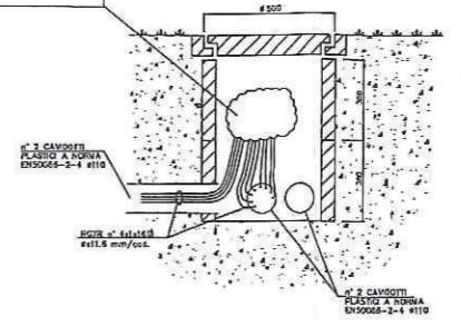
TIPICO INDICATIVO DERIVAZIONE IN POZZETTO
