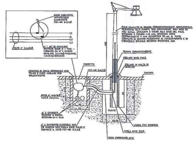
TIPICO INDICATIVO INSTALLAZIONE APPARECCHIO ILLUMINANTE "GUZZINI ILLUMINAZIONE" SISTEMA "CITY-WOODY" h 4 m
